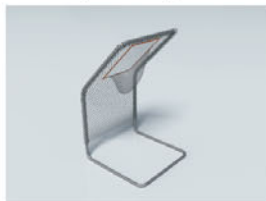
practice_net_2
